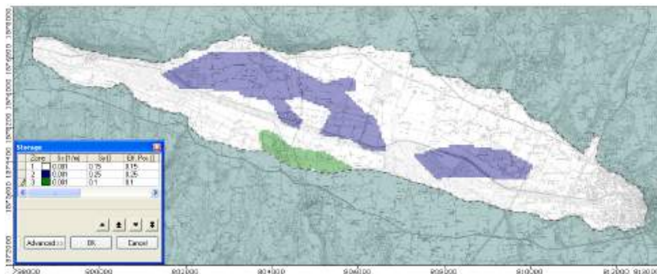
FIGURE 3.22 – Zones de coefficients d'emmagasinement obtenues à l'issue du calage.
