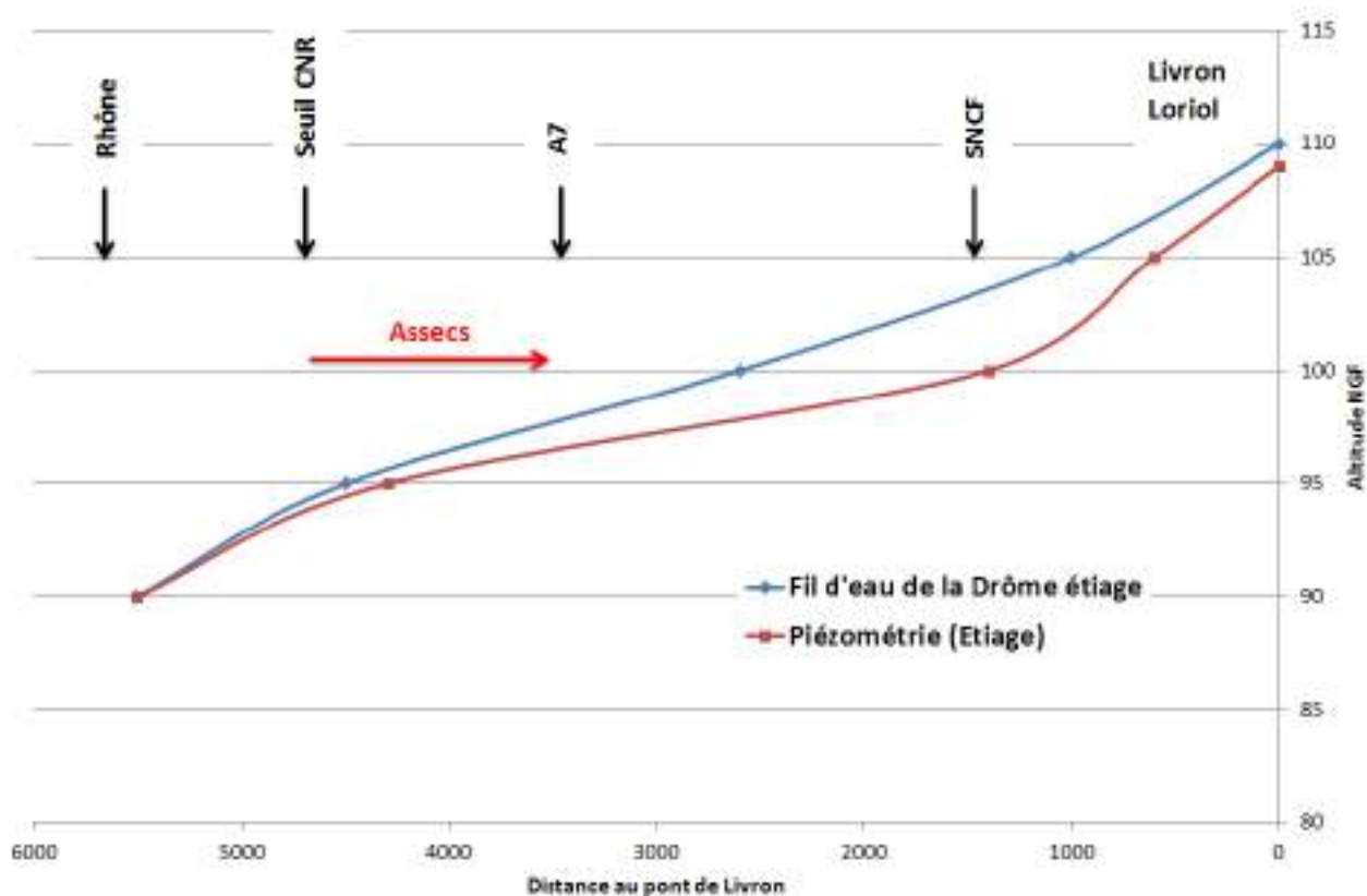
FIGURE 3.49 – Coupe présentant la ligne d'eau de la Drôme et la piézométrie des alluvions en période d'étiage (source relevés LIDAR 2010, et piézométrie de août 1996 (Géo+, 1997). La piézométrie est issue de la carte piézométrique interprétée de Géo+ à partir de données ponctuelles et non nivelées, situées à une distance significative du cours d'eau).
