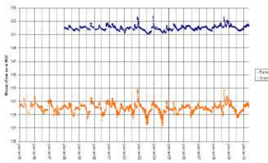
FIGURE 1.11 – Chronique piézométrique des piézomètres d'Alex et de Grane entre 1995 et 2010 (Données DIREN)
