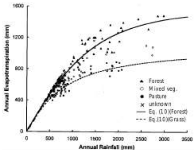
FIGURE 3.59 – Evapotranspiration annuelle en fonction de la précipitation annuelle pour des couverts forestiers et des couverts de paturages (d'après Zhang et al. [1999])
