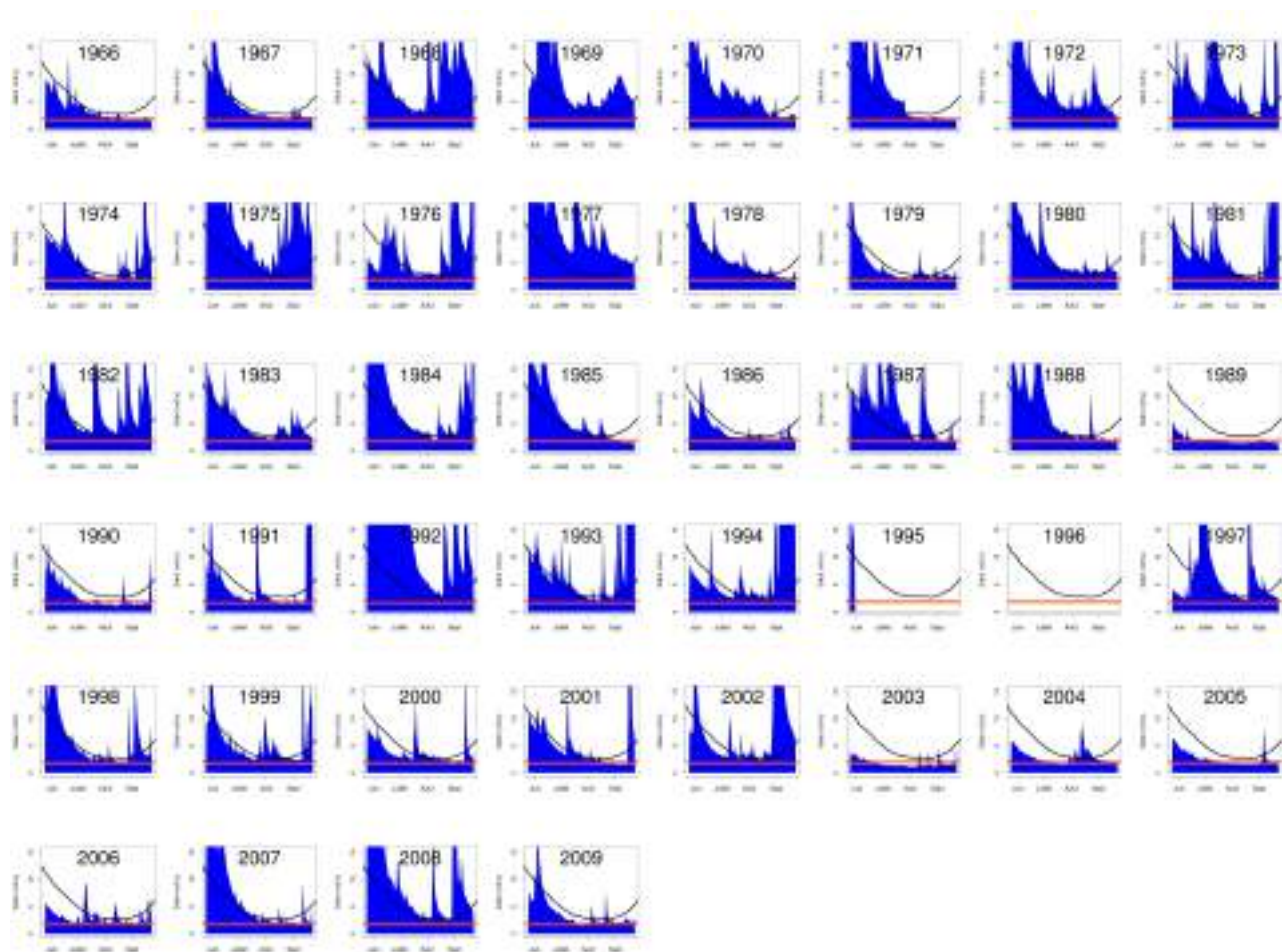
FIGURE 1.33 – Débits journaliers (en bleu) sur la période d'étiage (de juin à septembre) de la Drôme à la station hydrométrique de Saillans, pour les années 1966 à 2009. Le trait noir est le débit journalier médian sur la période d'existence de la période, lissée avec une moyenne glissante sur 15 jours. Le trait orange est la valeur du VCN_{3-5} (débit minimal moyenné sur 3 jours de période de retour quinquennale)- NB : on ne dispose pas de données pour les années 1995 et 1996.
